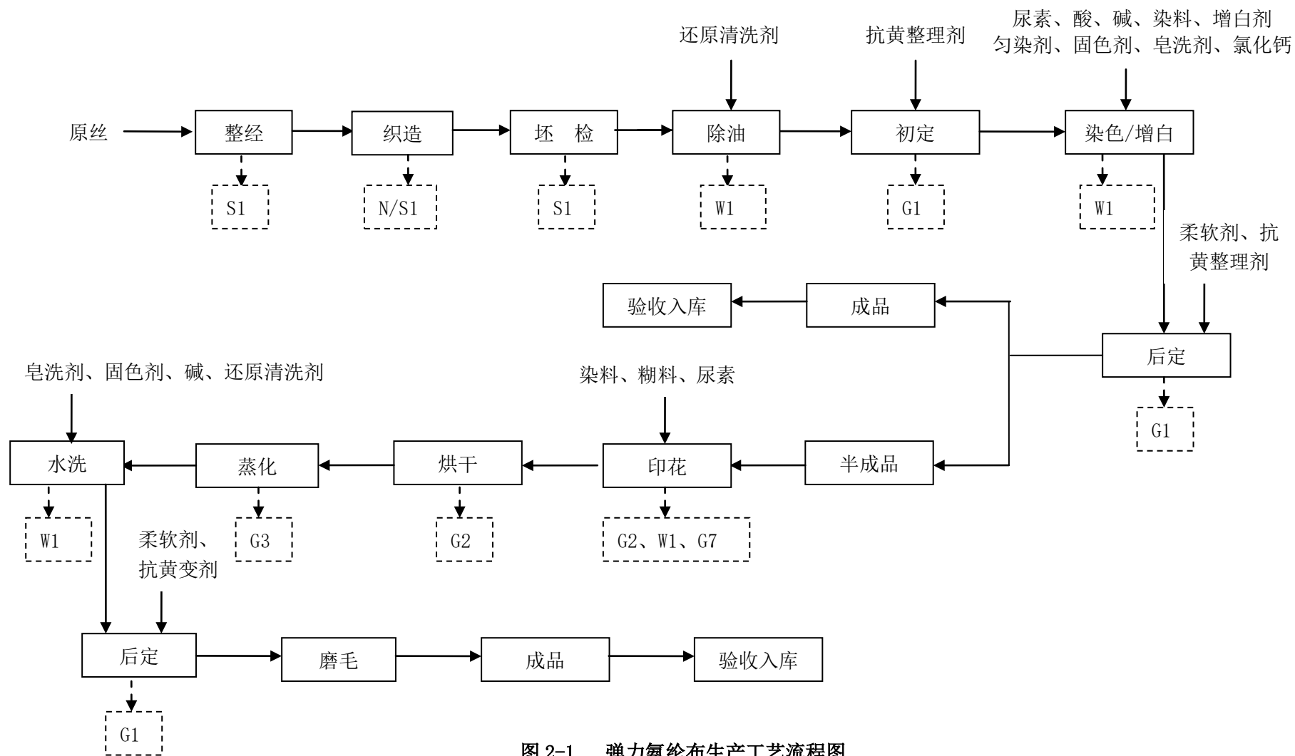
图 2-1 弹力氨纶布生产工艺流程图
